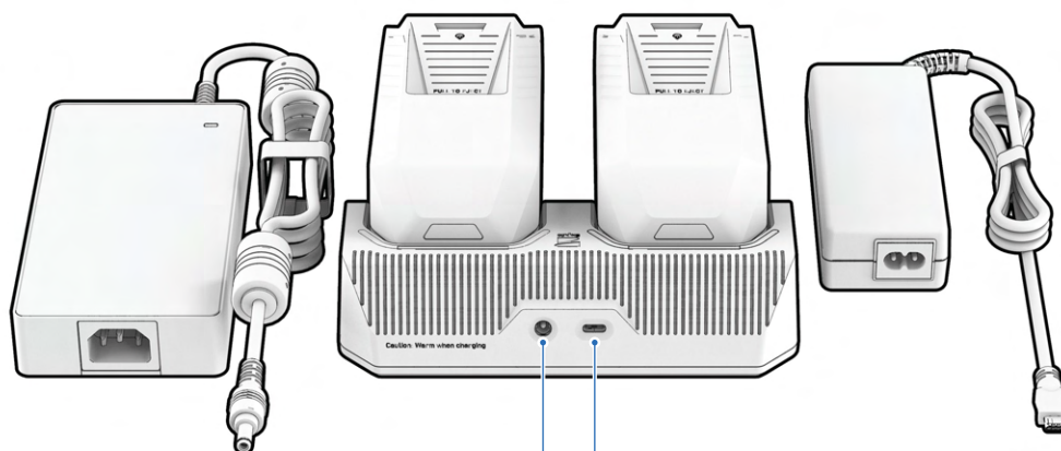
Fuente de alimentación rápida de 230 W
